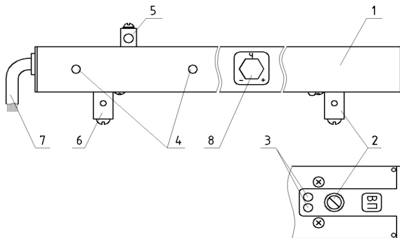
Рисунок 1.3 Конструкция ПРМ.
